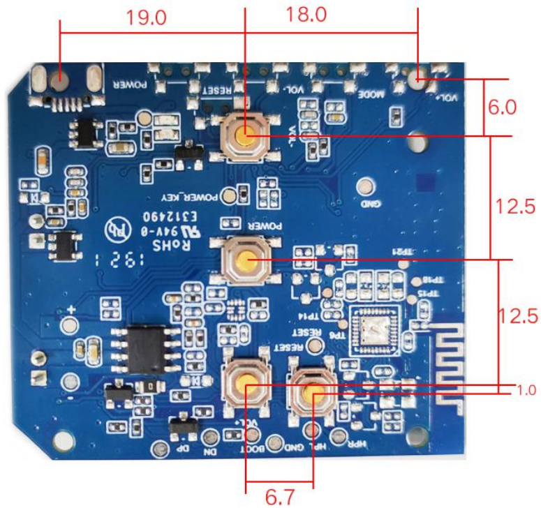
尺寸图-背面（单位：mm，正视图）
