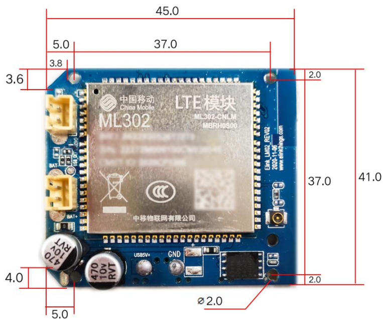
尺寸图-正面（单位：mm，正视图）
