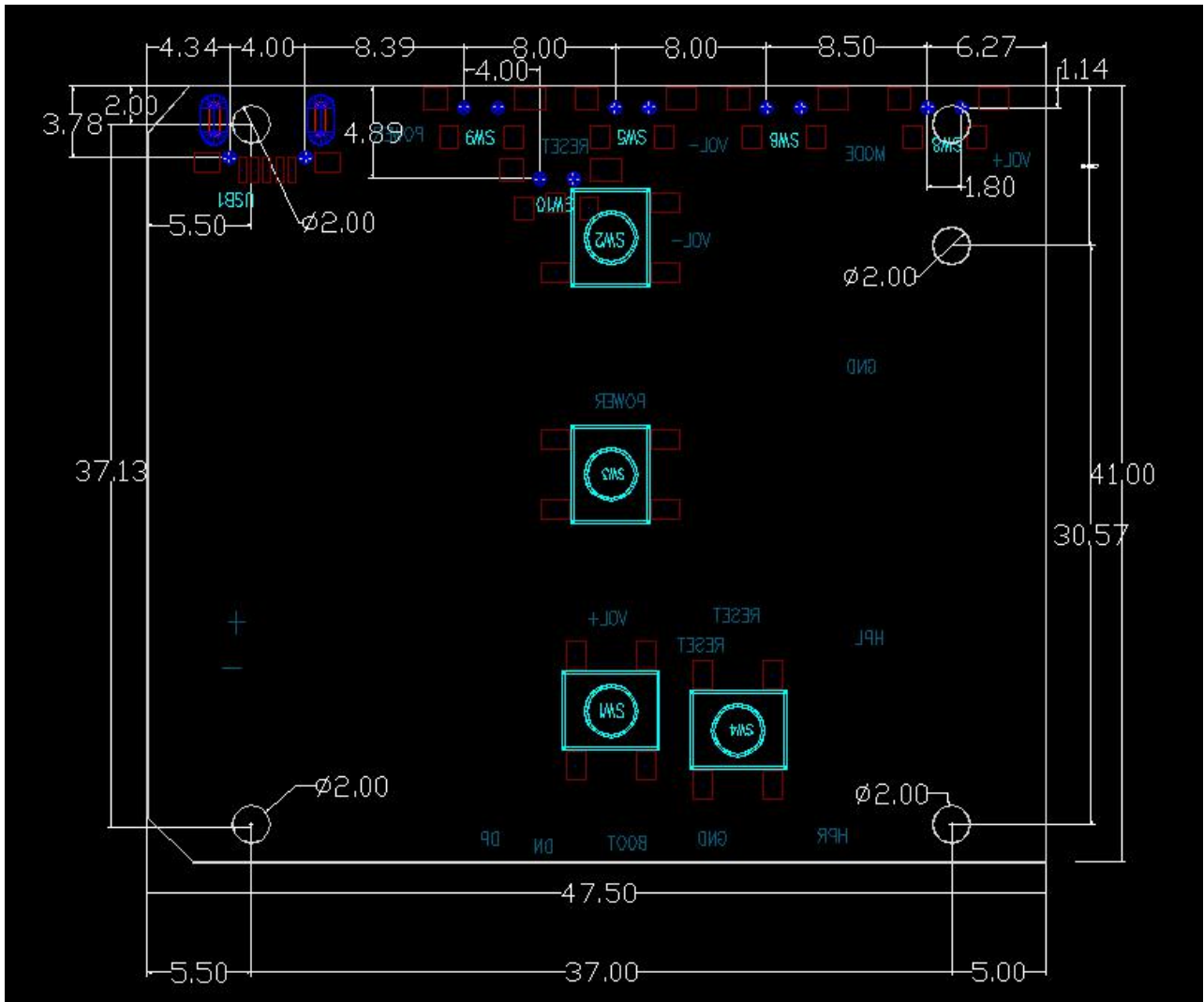
尺寸图-背面（单位：mm，正视图）
