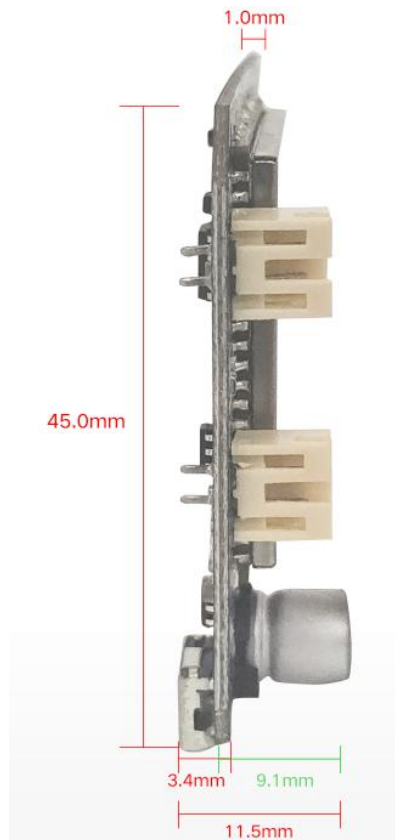
LM02 封装尺寸- (单位: mm , 侧视图)
