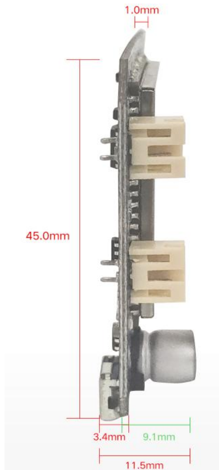
LM02 封装尺寸-（单位：mm，侧视图）
